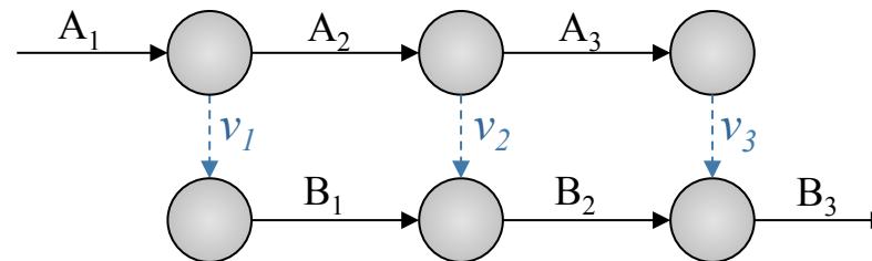
Representación PERT
